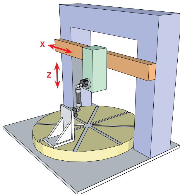
Типовой 2-координатный вертикальный токарный станок с VTL-адаптером на резцедержателе
